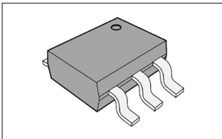
Рис. 10. Корпус SOIC-6 (4,6x6,3 мм)
