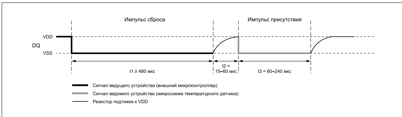
Рис. 1. Временная диаграмма инициализации микросхемы
