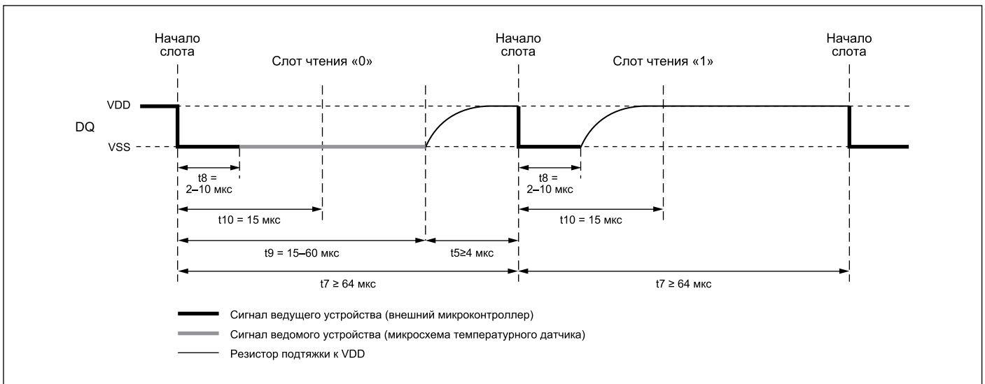
Рис. 3. Временная диаграмма чтения данных
